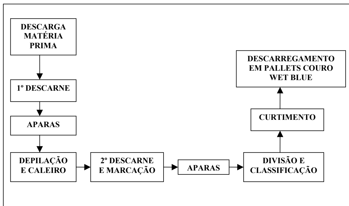
Figura 8 : Fluxograma da Produção
